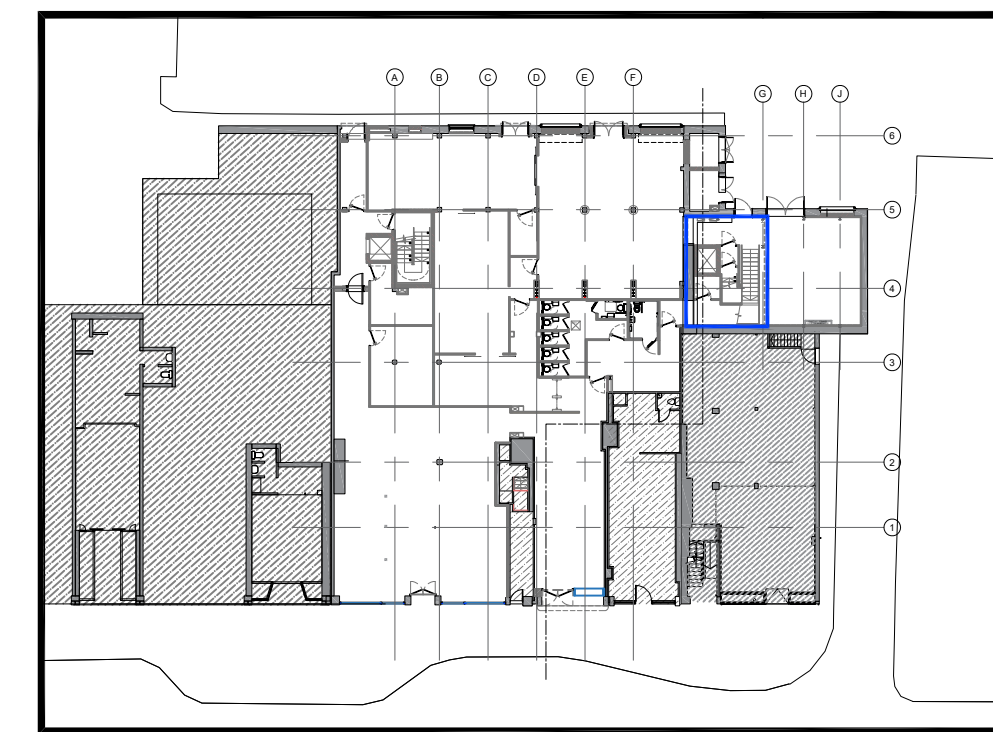
10 63.01 GFL_KEYPLAN SCALE: NTS
