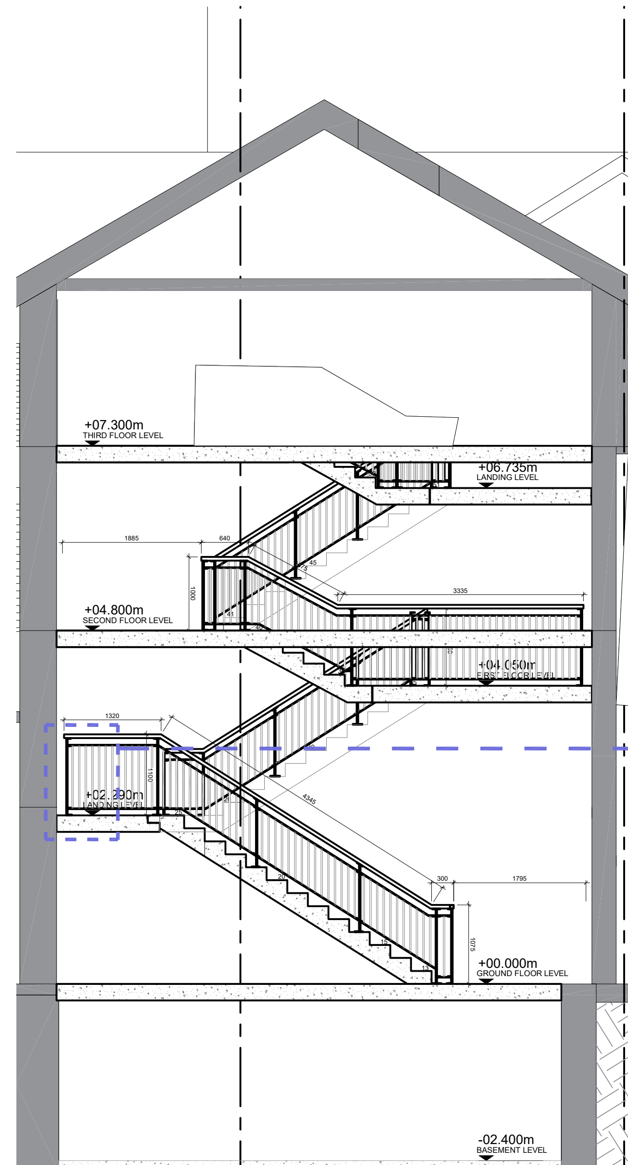
8 63.01 SECTION C-C SCALE: 1:50
