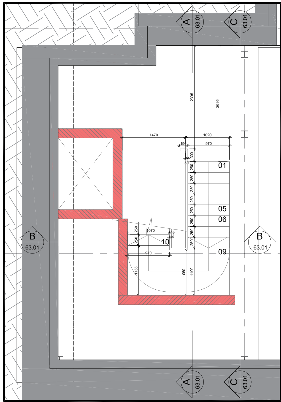
1 63.01 BASEMENT_KEYPLAN SCALE: 1:50
