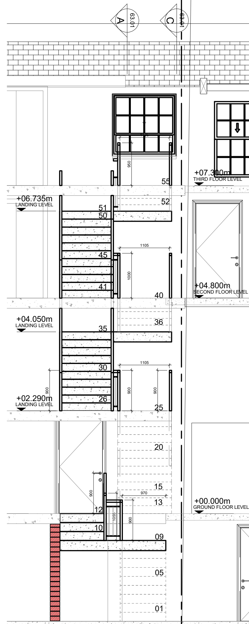
7 63.01 SECTION B-B SCALE: 1:50
