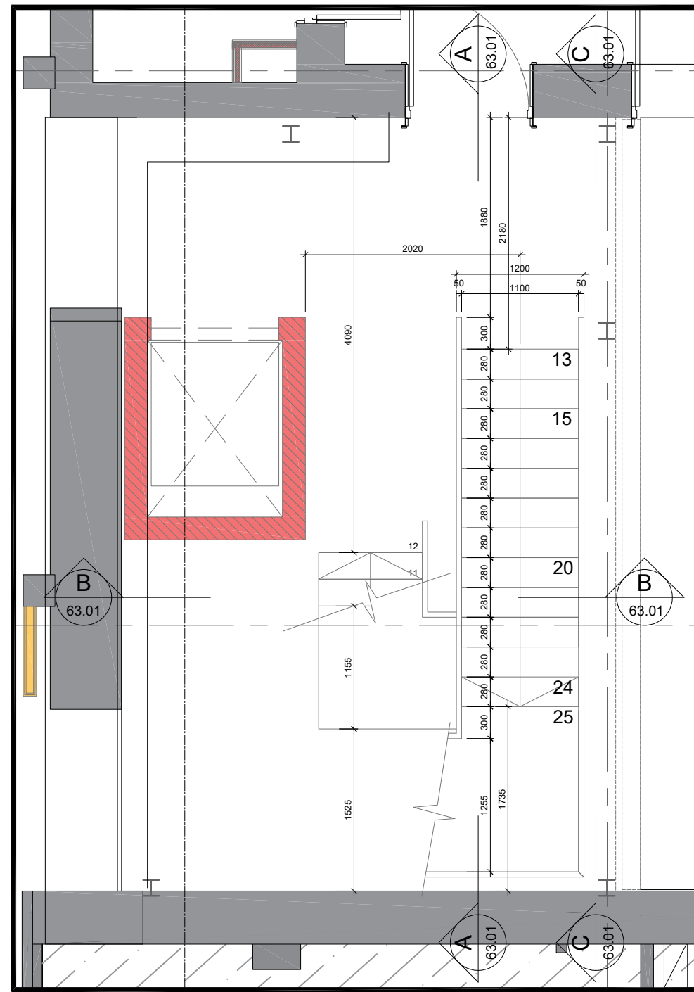
2 63.01 GFL_KEYPLAN SCALE: 1:50
