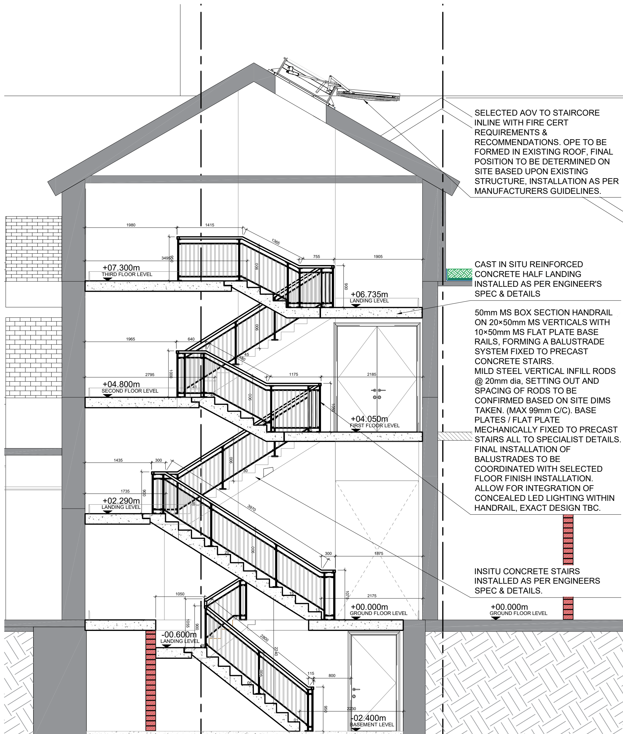
6 63.01 SECTION A-A SCALE: 1:50
