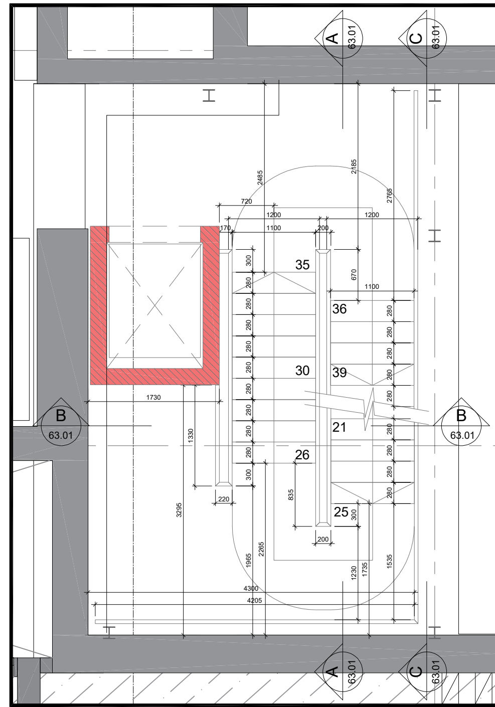
3 63.01 FIRST_FL_KEYPLAN SCALE: 1:50
