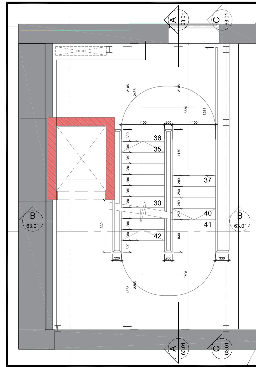
4 63.01 SECOND_FL_KEYPLAN SCALE: 1:50
